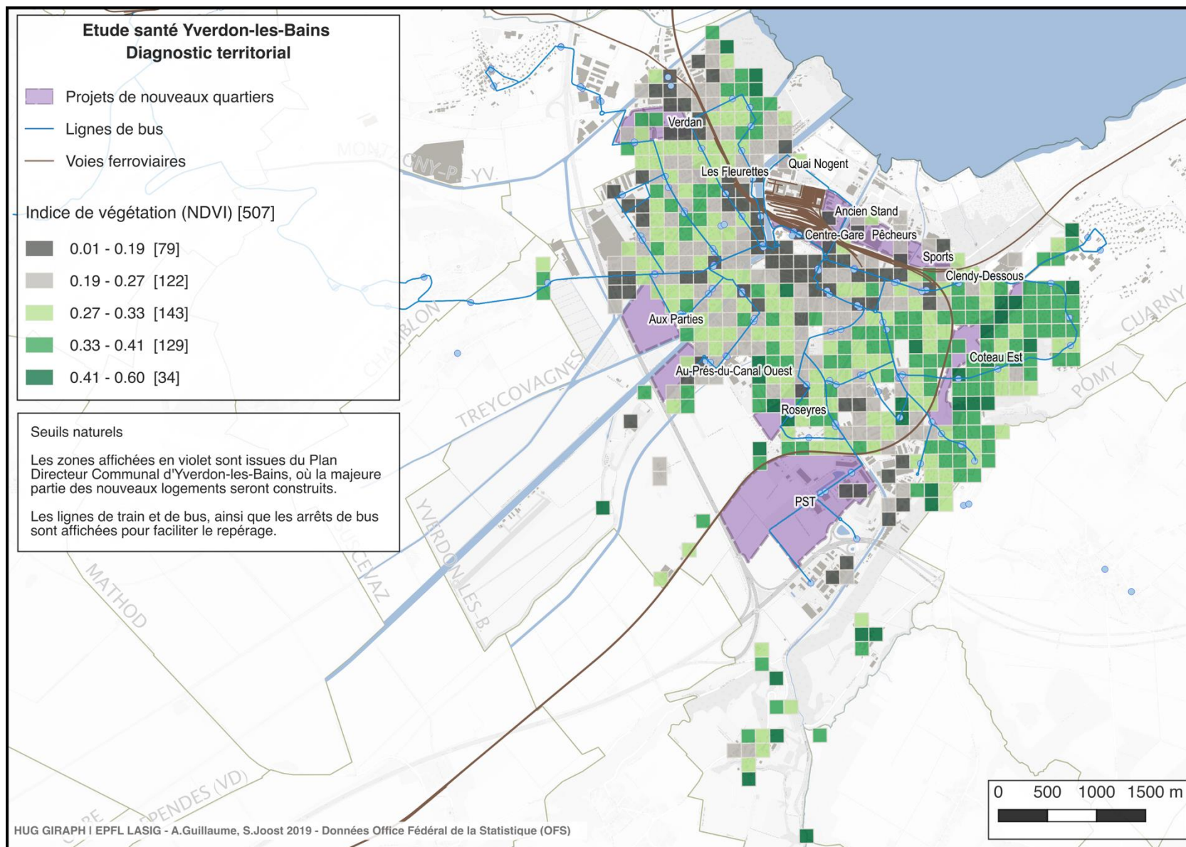
Figure 9 : NDVI (indice de végétation par différence normalisée) (source : LandSat 8, U.S. Geological Survey).
