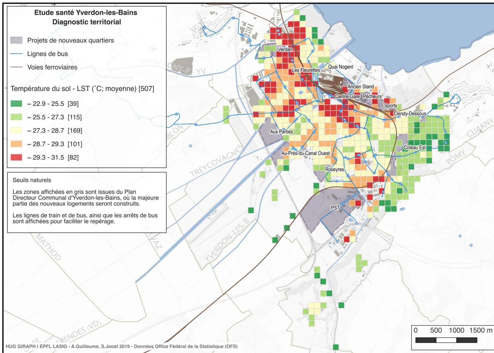
Figure 10 : Températures moyenne du sol (source : LandSat 8, U.S. Geological Survey).
