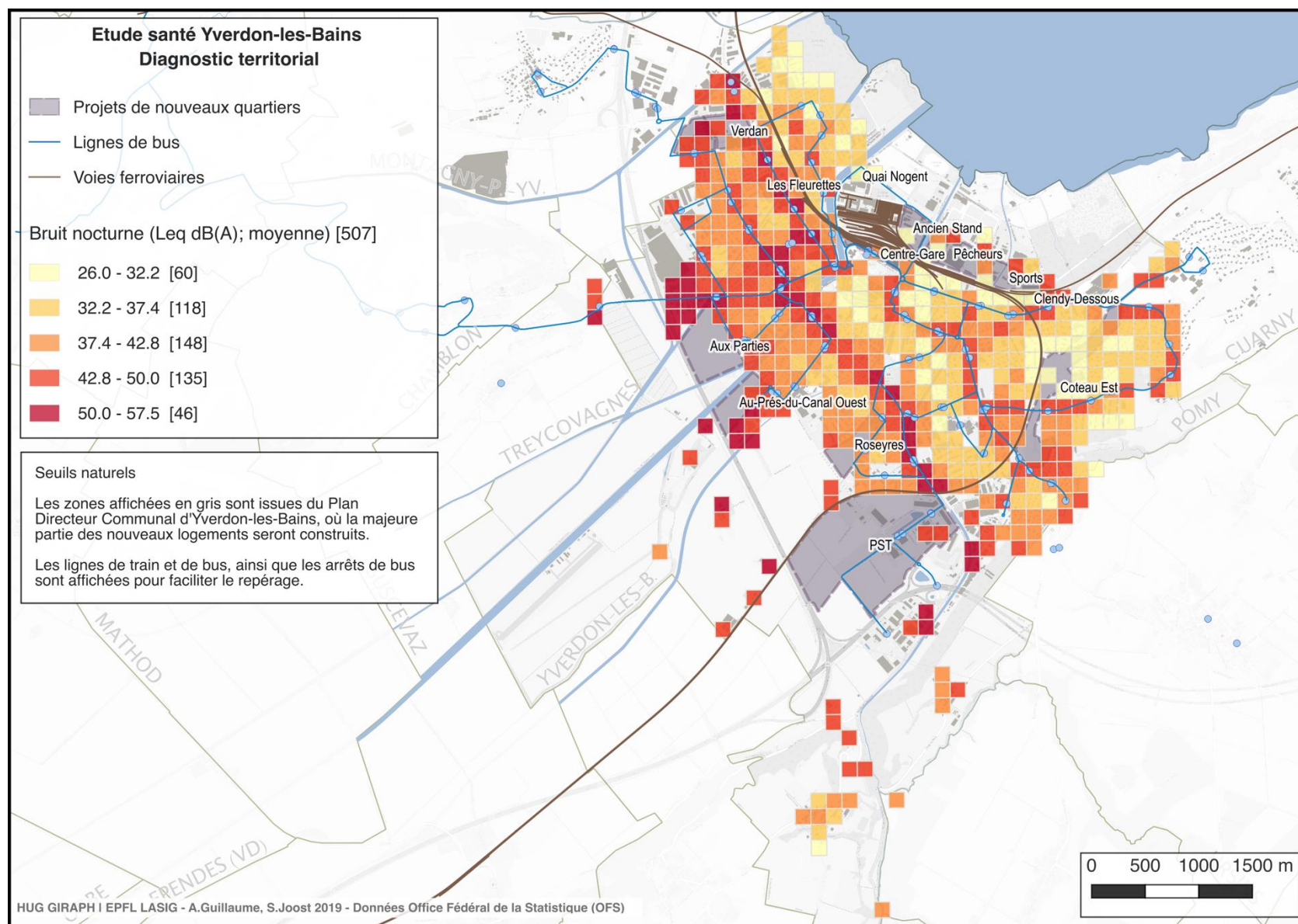
Figure 11 : Bruit routier nocturne.
